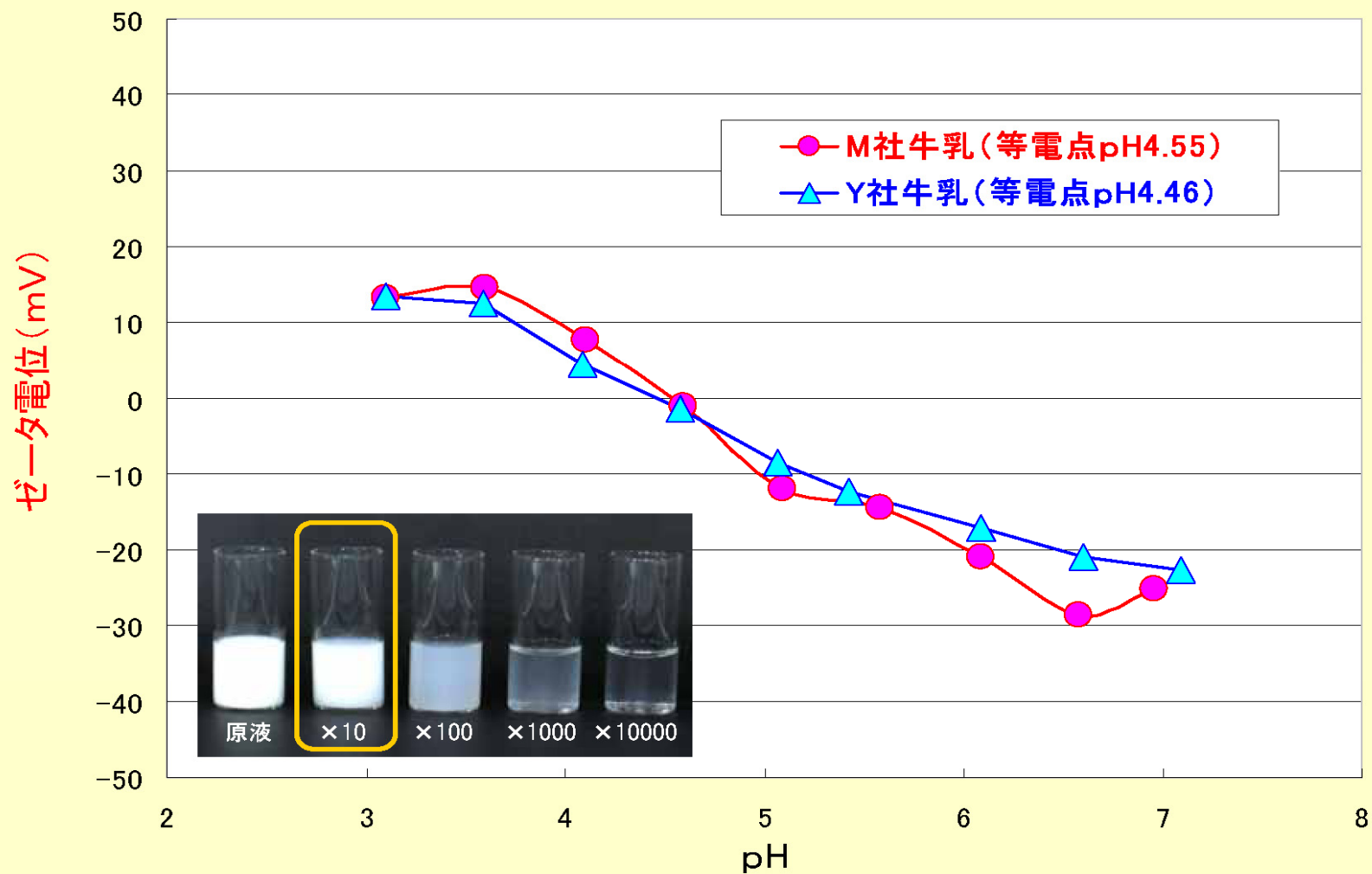
牛乳のゼータ電位のpH依存性
